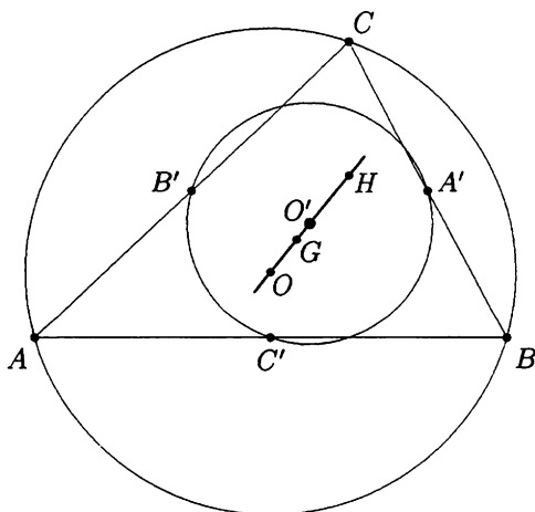
Figura 33: Recta d'Euler
